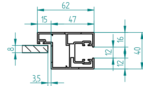
Schnitt A-A 1:2
