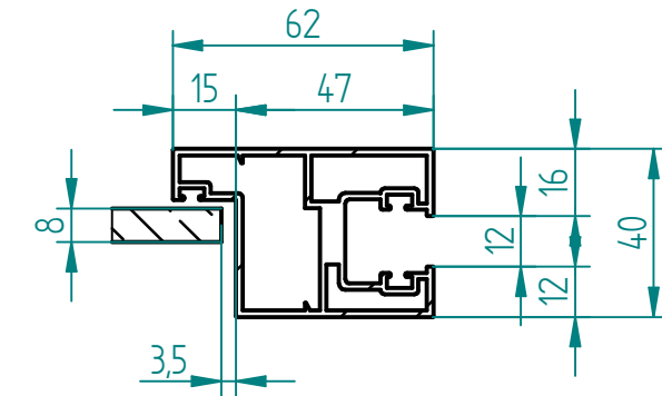
Schnitt A-A 1:2
