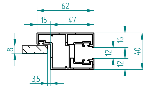
Schnitt A-A 1:2
