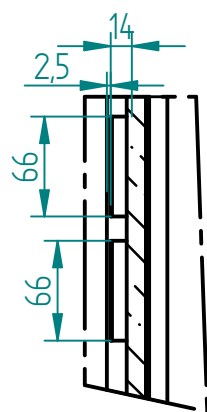
EINZELHEIT C
