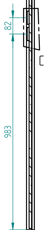
Schnitt B-B
