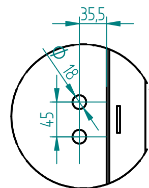
EINZELHEIT D
