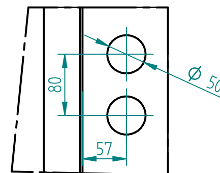
EINZELHEIT E
